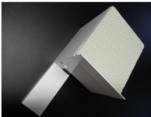
Vorbaurollladen SP mit Putzträger Kastengrößen SP 137, 165, 180, 205
