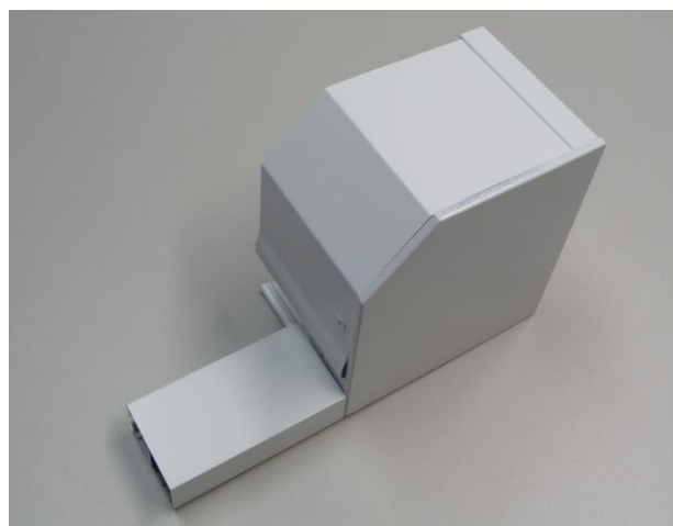
Vorbaurollladen SK mit sichtbaren Kasten (vordere Kante abgeschrägt) Kastengrößen SK 137, 165, 180, 205
